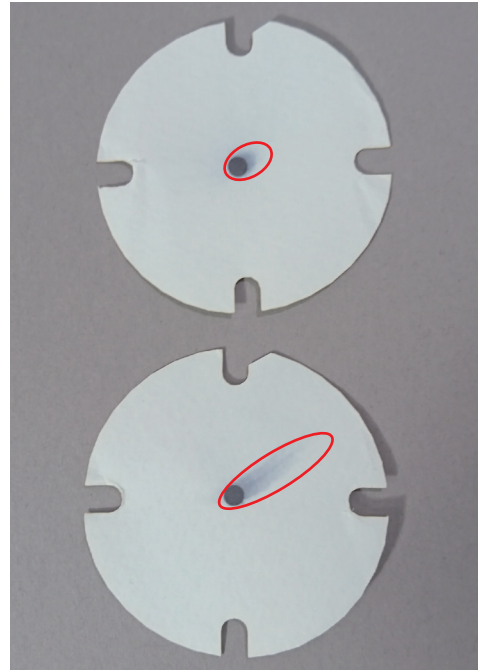
0.1cm と 0.7cm/min のテーリング比較
